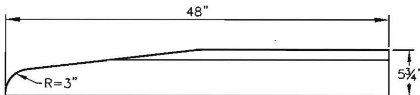
ELEVATION
